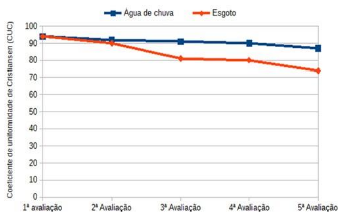
Figura 5. Prática de avaliação do coeficiente de uniformidade de Christiansen (esquerda); resultados do CUC para os sistemas irrigados com esgoto tratado e com água de chuva (direita).
